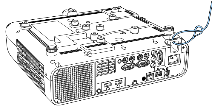
Bei Installation der Kabelabdeckung (EB-L265F)
